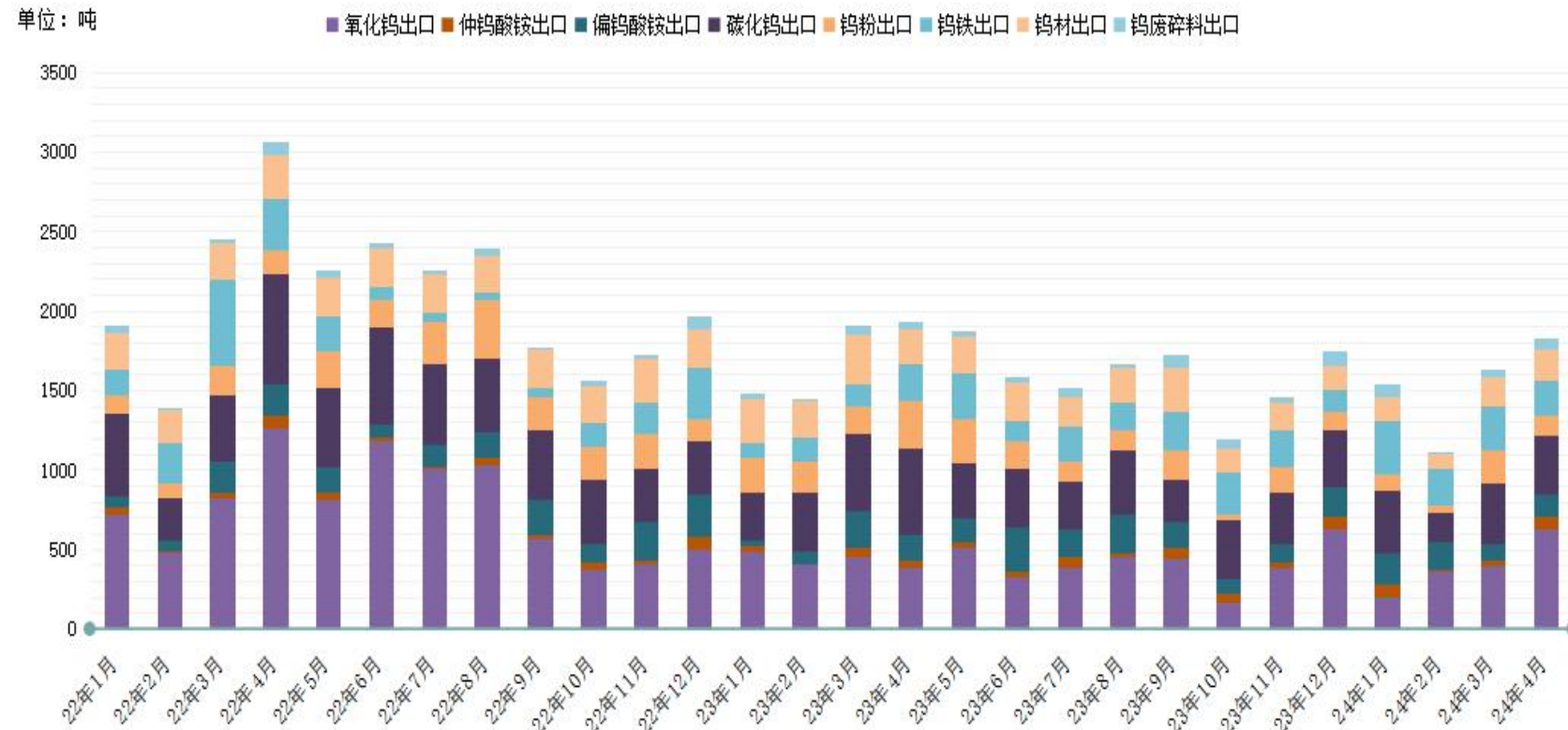
钨钼云商：2022-2024年中国钨产品出口数据图
